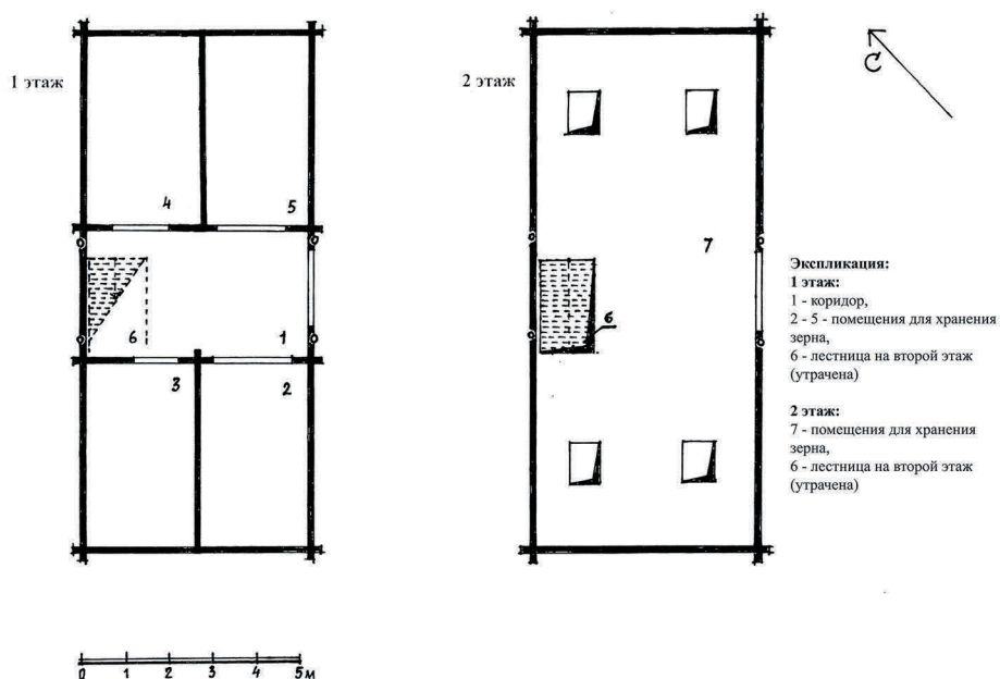
Рис. 2. Амбар-магазин (южный фасад), с. Ворзогоры, Онежский р-н, конец XIX – начало XX в. (фото Т. Жигальцовой, 2018 г.); план амбара-магазеи. Руководитель научного проекта, д. культ. А. Б. Пермиловская. Научная информация Т.В. Жигальцовой. Обмеры Т.В. Жигальцовой, А.А. Усова. Камеральная обработка архитектора Н.А. Подобиной, 2018 г.
